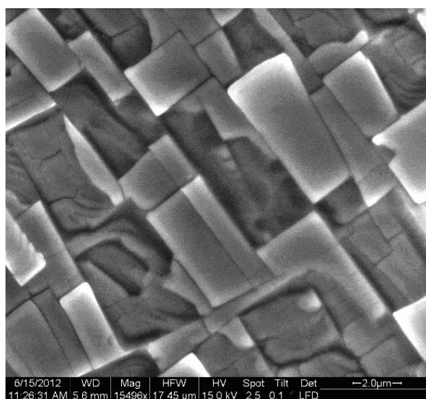
Рис. 2. Микрофотография поверхности диоксида циркония при сканировании лазерным пучком ArF-лазера при плотности энергии в импульсе 0,18 \text{ Дж/см}^2 с шагом между пятнами облучения 20 мкм и частотой повторения импульсов f = 2 \text{ Гц} .
