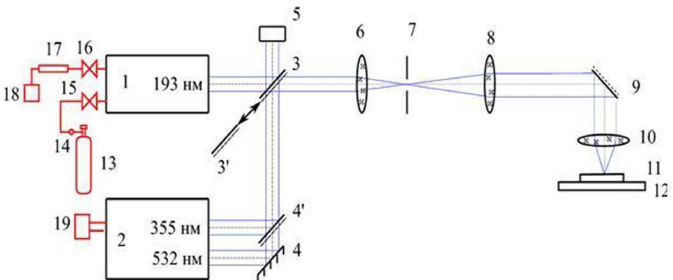
Рис. 1. Схема лазерной установки для микро- и наноструктурирования.
