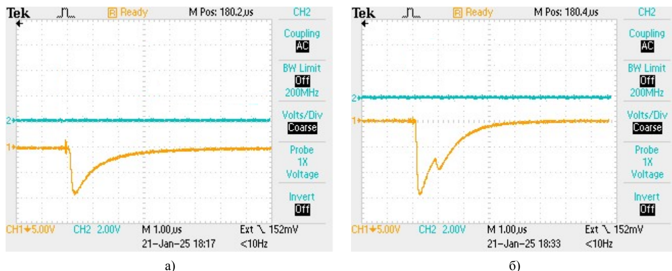
Рис. 2. Характерные осциллограммы тока разряда в аperiодическом режиме протекания тока при давлении p = 3 атм и R_b = 2 \Omega : а) – U_0 = 8 кВ, б) – U_0 = 11 кВ
