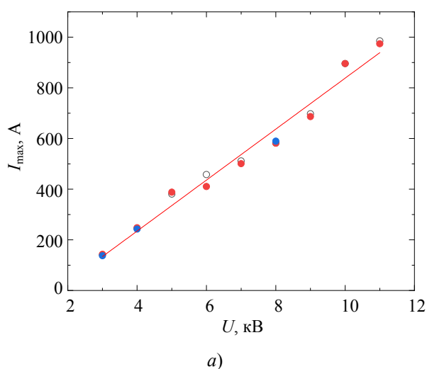
Рис. 3. Амплитудные значения тока разряда в аperiодическом режиме при разных условиях эксперимента: а) R_b = 2 \Omega , p = 1 атм, б) R_b = 52 \Omega , p = 1 атм и 3 атм.
