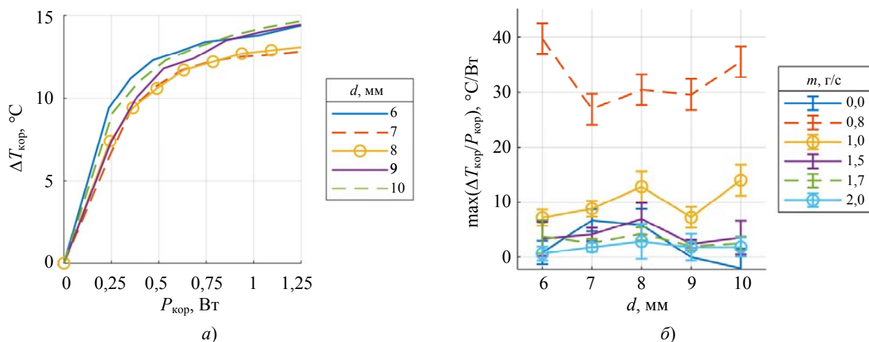
Рис. 4. Зависимость перепада температуры \Delta T_{\text{кор}} от мощности КР P_{\text{кор}} для различных значений ширины канала d при фиксированном расходе вентилятора m = 0,8 г/с (а) и максимального соотношения \Delta T_{\text{кор}}/P_{\text{кор}} при различных d и m (б)
