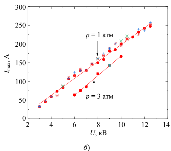
Рис. 3. Амплитудные значения тока разряда в аperiодическом режиме при разных условиях эксперимента: а) R_b = 2 \Omega , p = 1 атм, б) R_b = 52 \Omega , p = 1 атм и 3 атм.
