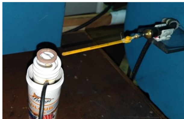
Рис. 1. Фотография системы диэлектрическое кольцо на спиральной лампе. Справа расположен зонд магнитного поля
