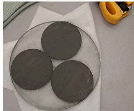
Рис. 2. Иллюстрация решения двумерной задачи упаковки для диска-носителя диаметром 112 мм и пластин InSb диаметром 50,8 мм (а) и фото приклеенных на диск-носитель пластин InSb (б)
