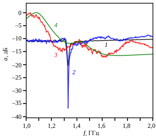
Рис. 4. Резонансные спектры магнитного поля для кольца и прямого проводника длиной полуолны (115 мм): 1 (черный) – расчет, одиночное диэлектрическое кольцо, f_0 = 1,350 ГГц, a_0 = -11,832 дБ; 2 (синий) – эксперимент, одиночное диэлектрическое кольцо f_0 = 1,331 ГГц, a_0 = -28,675 дБ; 3 (красный) – эксперимент, кольцо с проводником; 4 (зеленый) – расчет, кольцо с проводником
